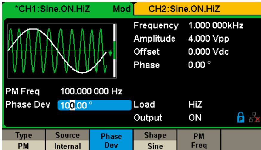
Abbildung 43: Bedienschnittstelle PM-Modulation
