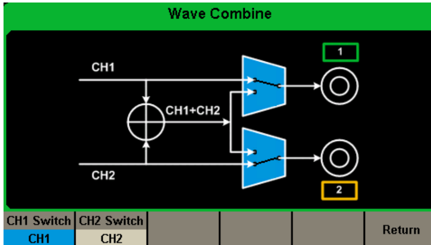
Abbildung 79: Bedienschnittstelle Signalformen-Kombination
