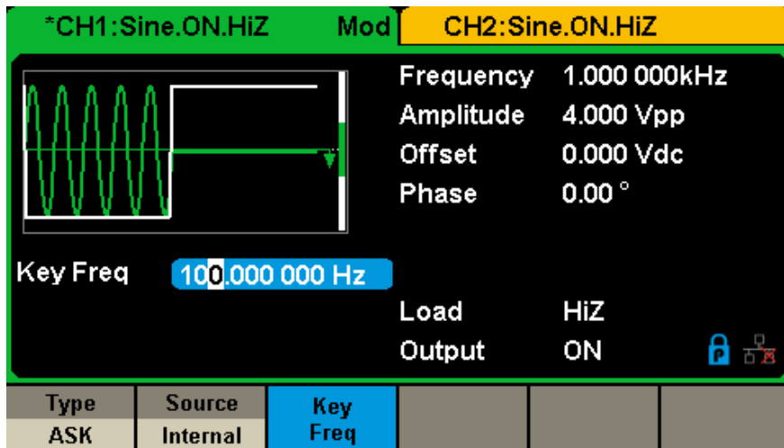
Abbildung 45: Bedienschnittstelle ASK-Modulation
