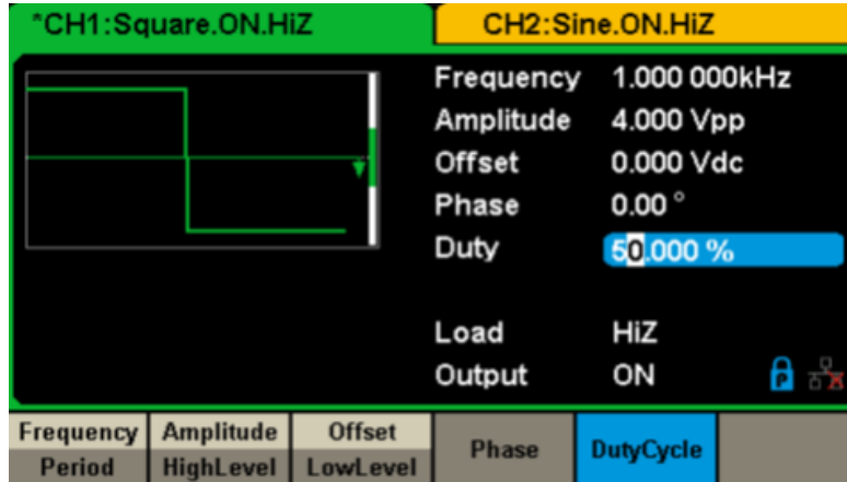
Abbildung 25: Bedienschnittstelle Rechtecksignal-Einstellungen
