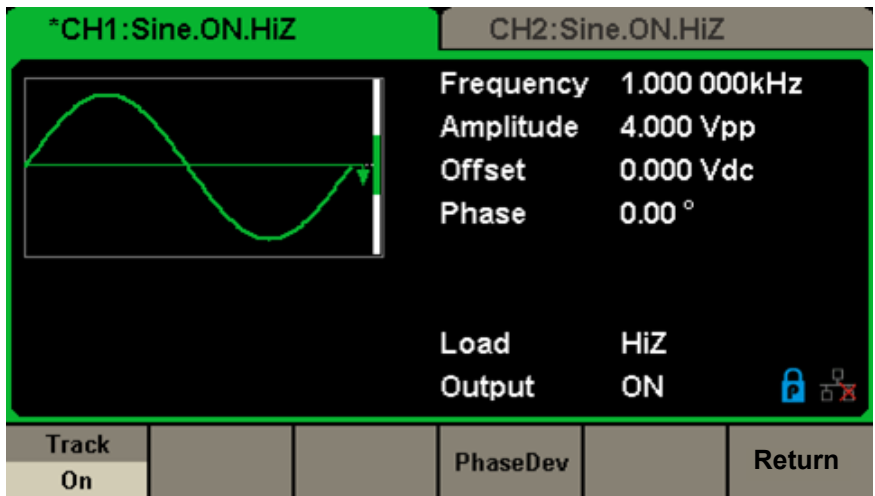
Abbildung 82: Bedienschnittstelle Tracking
