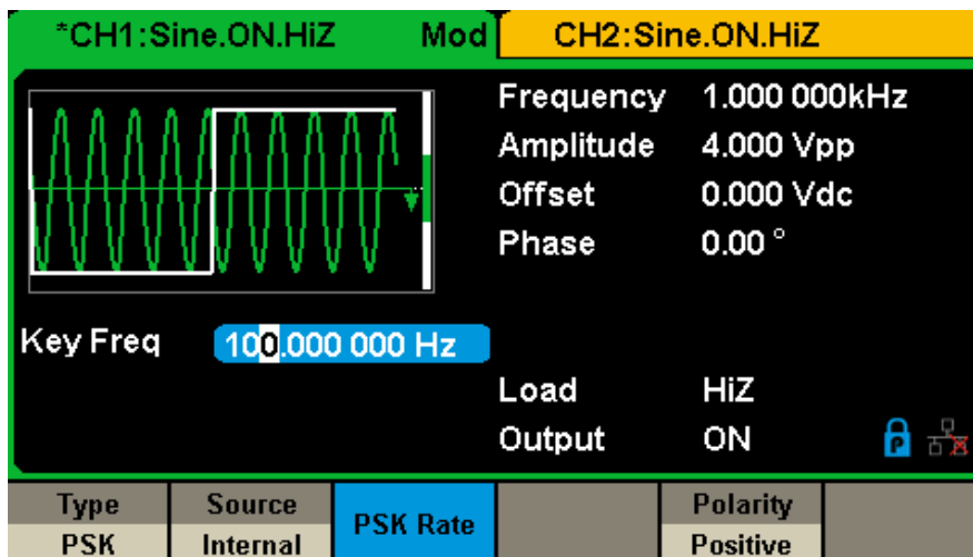
Abbildung 46: Bedienschnittstelle PSK-Modulation
