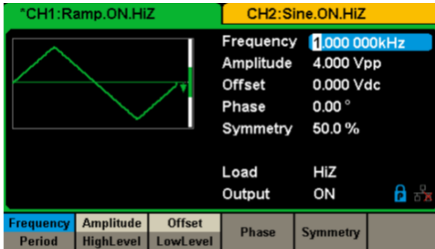
Abbildung 8: Bedienschnittstelle Dreiecksignal
