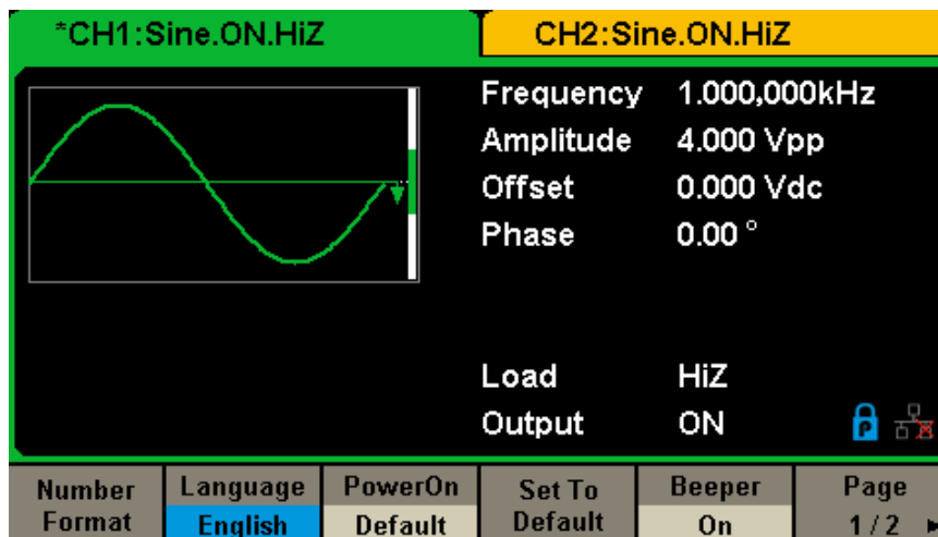
Abbildung 66: Schnittstelle auf Englisch
