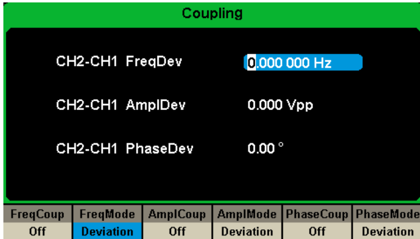
Abbildung 81: Schnittstelle Kanalkopplung
