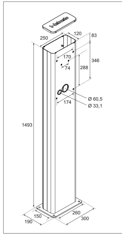
Fig. 04: Stand dimensions
