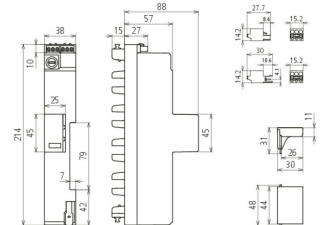
Maßbild DSH ZP B2 SG TNS 255
