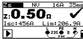
Abbildung 5.25: Beispiel Schleifenimpedanzmessung
