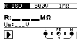
Abbildung 5.5: Isolationswiderstand
