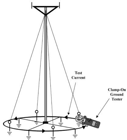
Abb. 24: Mobilfunkmast – Beispiel einer falsch eingesetzten Anwendung
