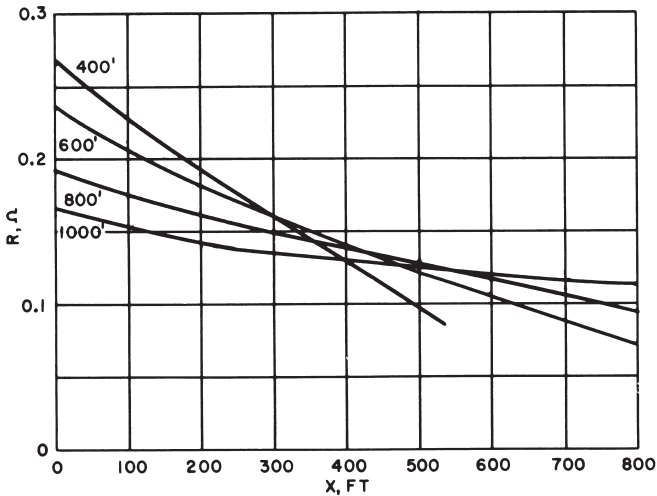
Abb. 30: Schnittkurven für Abb. 29 Die Mitte des Dreiecks, das durch die Überschneidung in Abb. 30 gebildet wird, zeigt einen Erdungswiderstand von 0,146 \Omega
