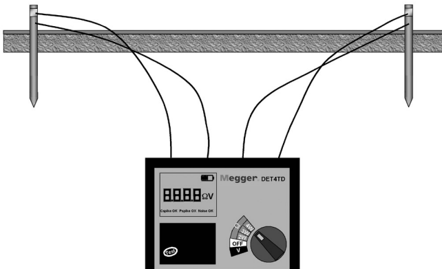
Abb. 34: Durchführung einer Zweipunktmessung
