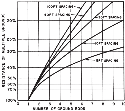
Abb. 18: Vergleichswiderstände von Erdungselektroden mit mehreren Stäben Ein Stab entspricht 100 % 9
