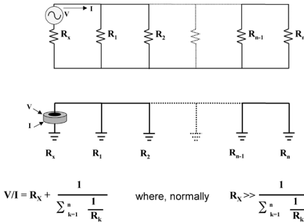
Abb. 22: Grundlegende Clamp-on-Verfahren für Erdungsprüfungen
