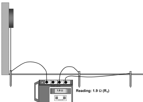
Abb. 25: Erdungswiderstandsmessungen
