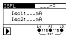
Abbildung 5.41: Erstfehler-Leckstrom ISFL
