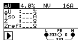
Abbildung 5.27: Spannungsfall
