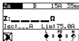
Abbildung 5.23: Schleifenimpedanz
