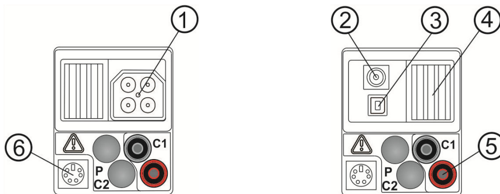
Abbildung 3.2: Anschlussfeld
