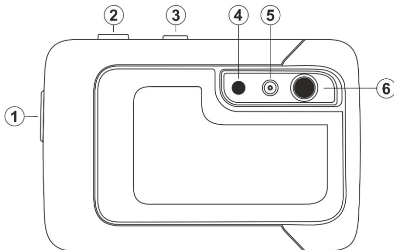
Abb. 2: Beschreibung der Vorderseite
