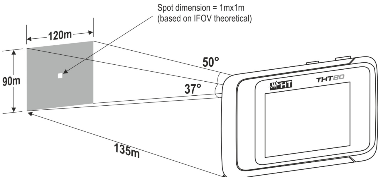
Abb. 50: Darstellung des Sichtfeldes FOV des Geräts
