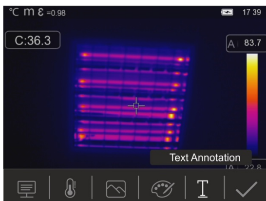
Abb. 47: Einfügen einer Textaufzeichnung auf dem Bild
