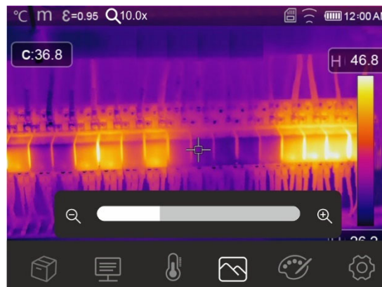
Abb. 38: Aktivierung des Zooms des Bildes
