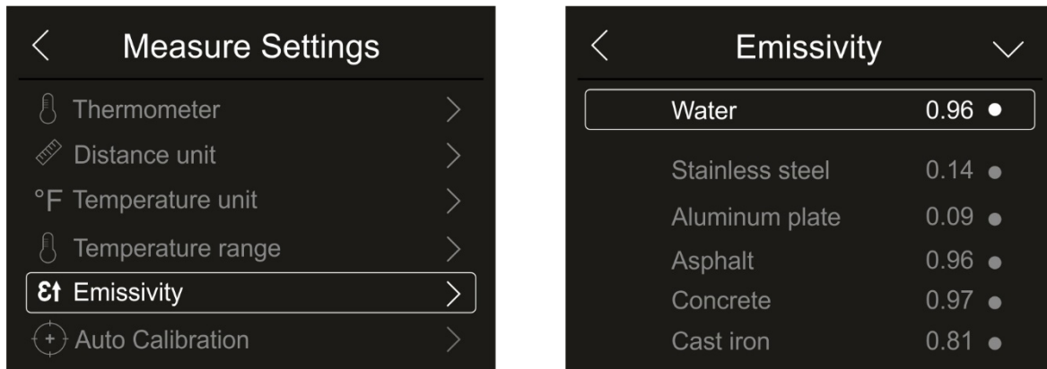
Abb. 28: Menü Einstellung der Emissivität
