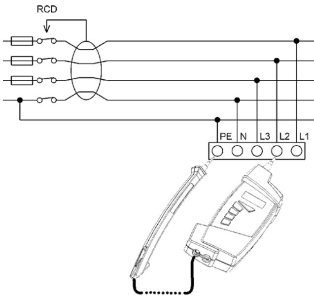
Bild 3.13 Anschlussbeispiel
