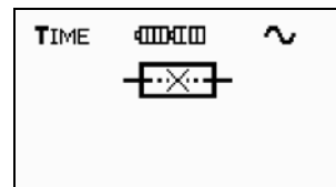
Bild 3.3 Anzeige der defekten Sicherung
